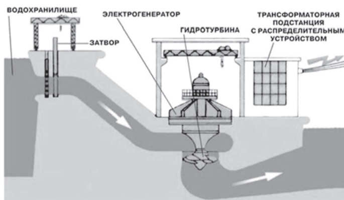
Принцип работы гидроэлектростанции
